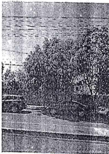
Árbol 4
