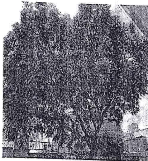
Árbol 8
