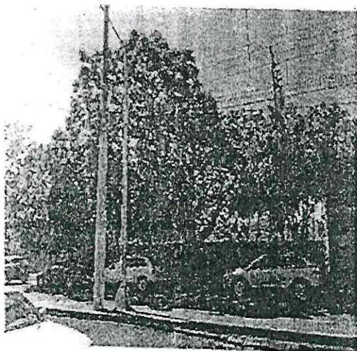
Árbol 1
