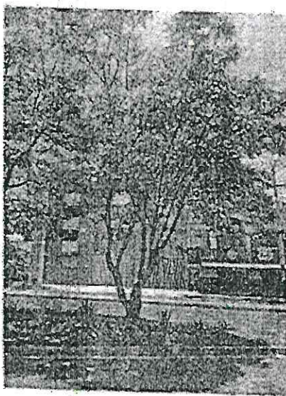
Árbol 6
