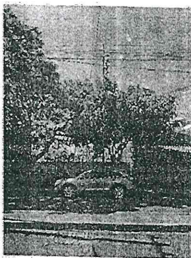
Árbol 2
